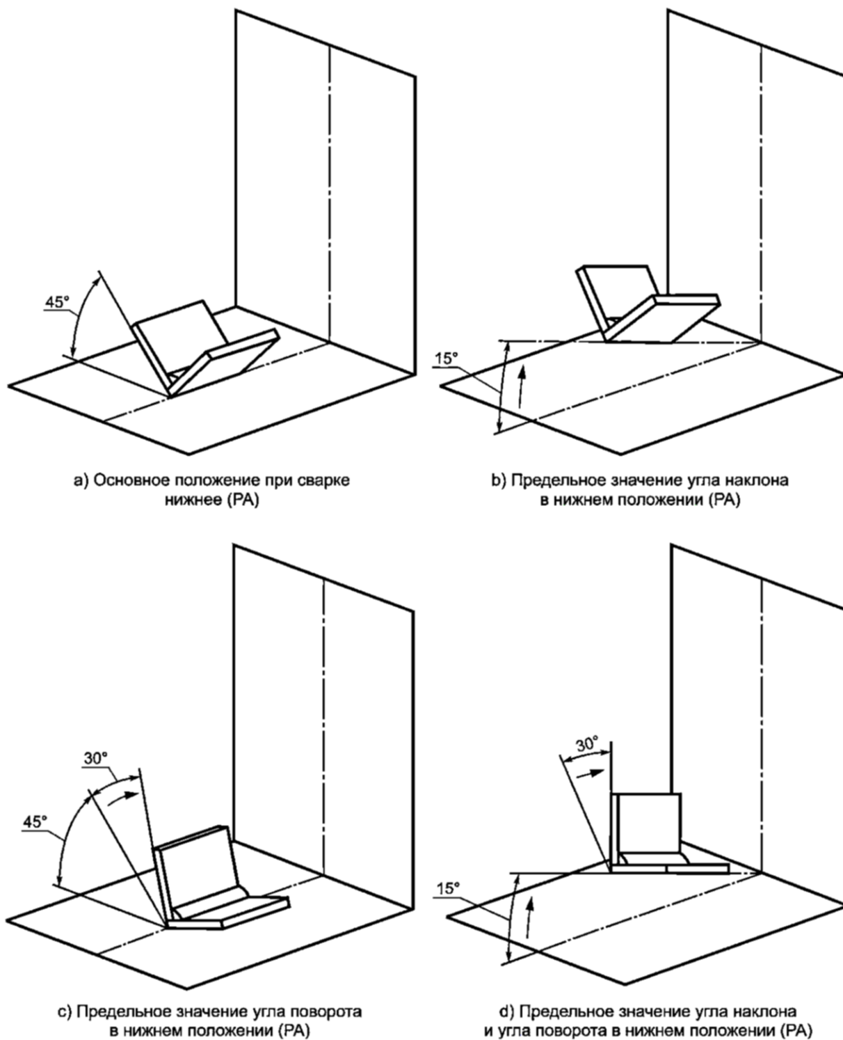
Рисунок А.5 — Предельные значения угла наклона и угла поворота для угловых швов в нижнем положении при сварке РА
